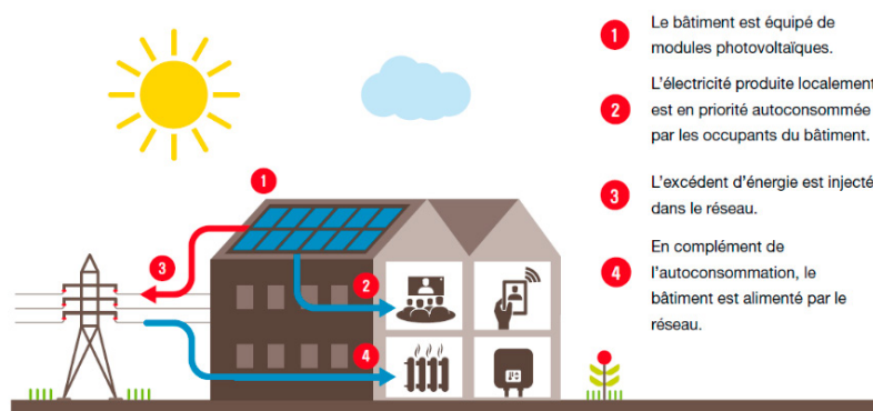
Production et consommation locale : principe de fonctionnement
